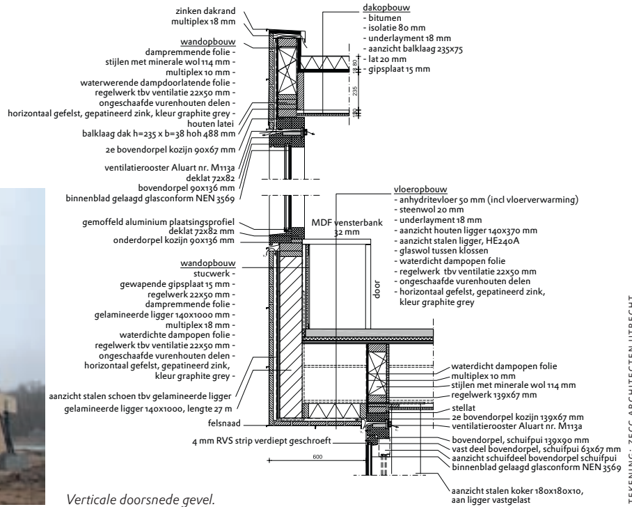
Verticale doorsnede gevel.
