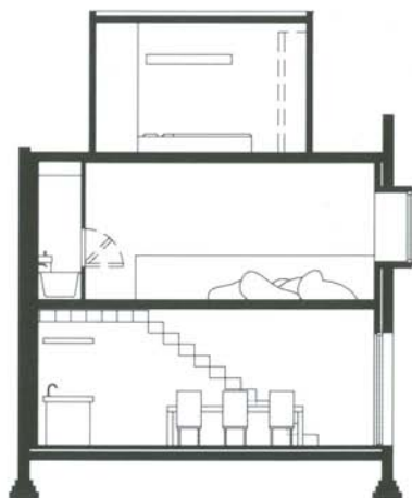
Section AA Sección AA
